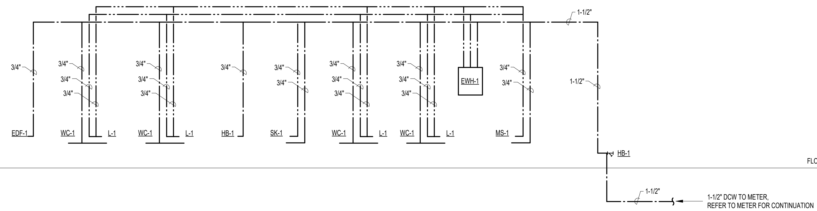
2 DOMESTIC WATER RISER DIAGRAM N.T.S.
